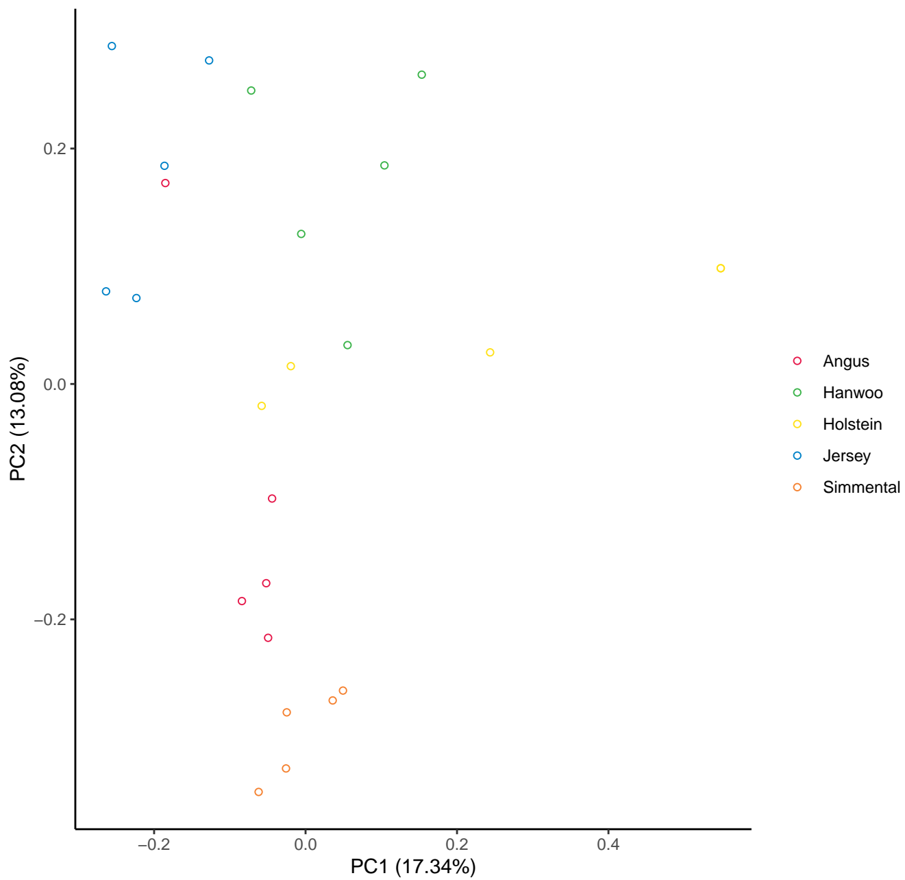
PCA analysis : 1-2
