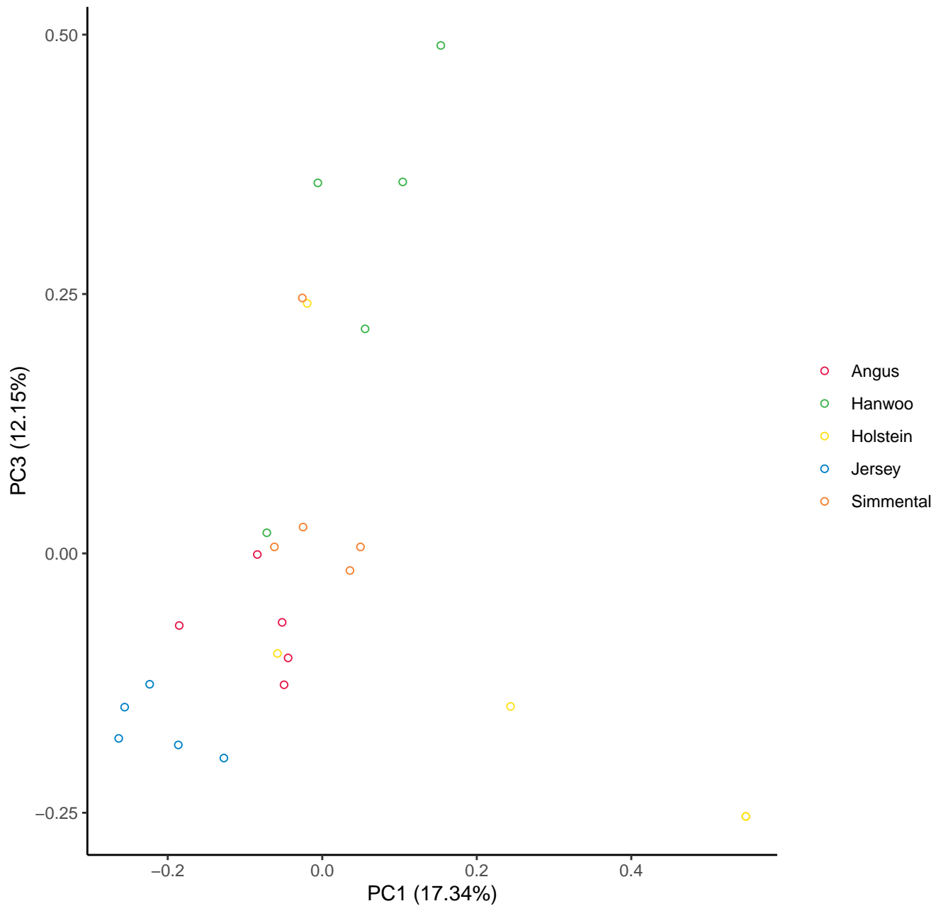
PCA analysis : 1-3
