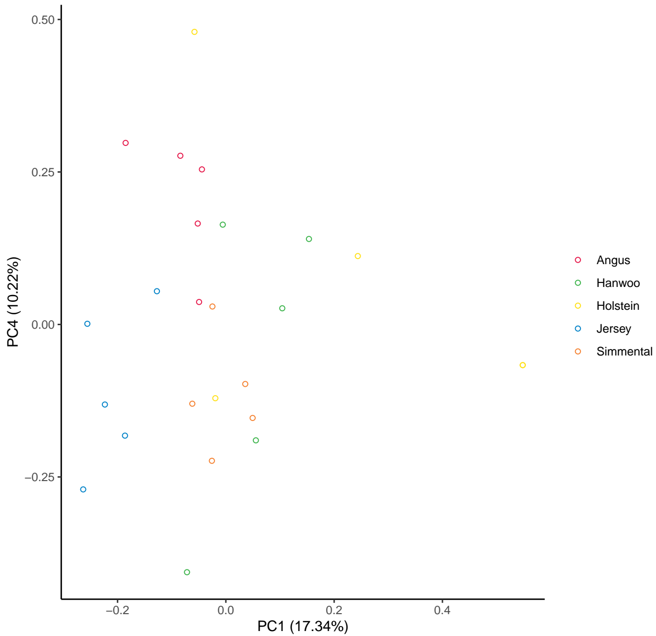
PCA analysis : 1-4
