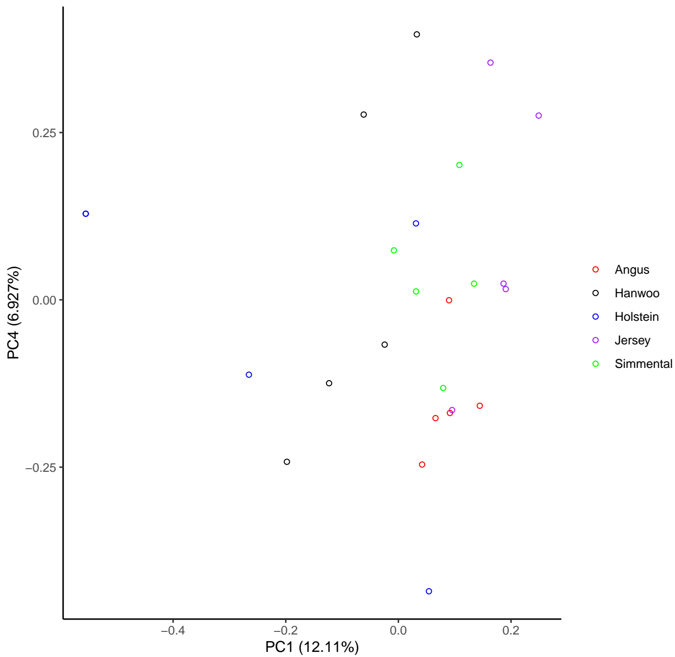
PCA analysis : 1-4
