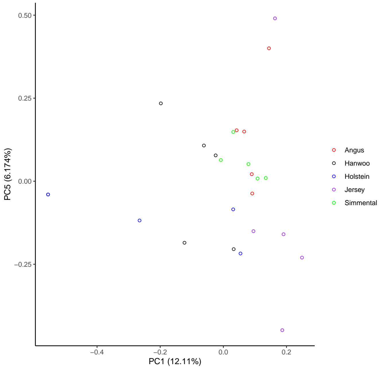
PCA analysis : 1-5
