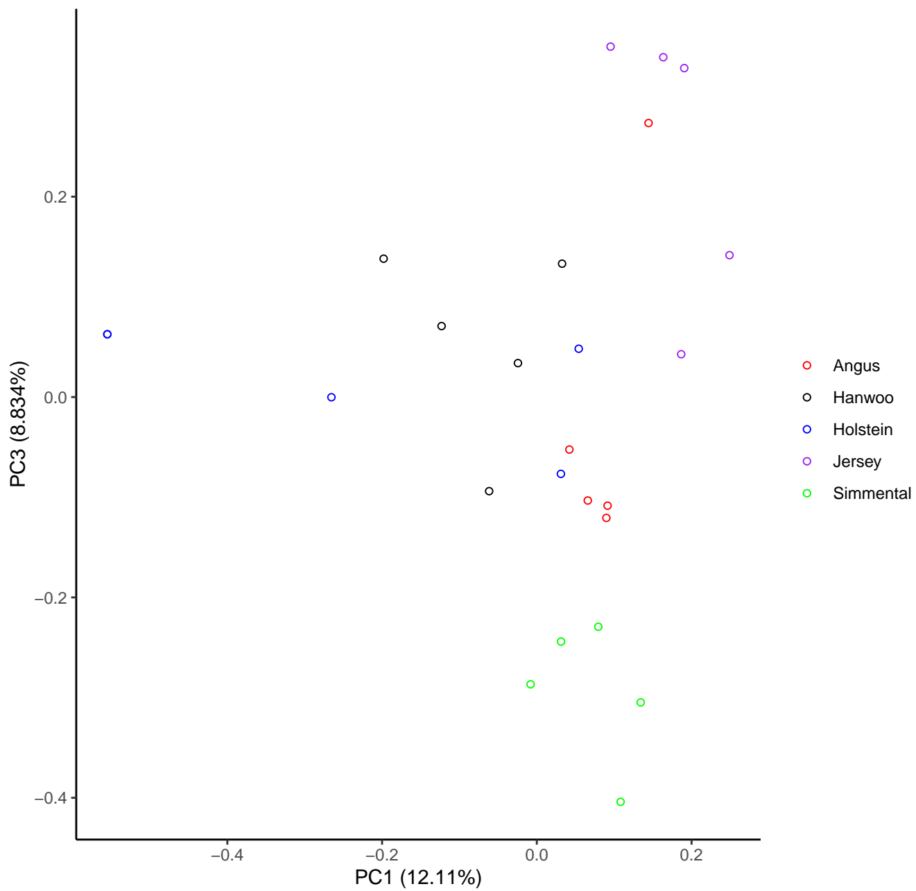
PCA analysis : 1–3
