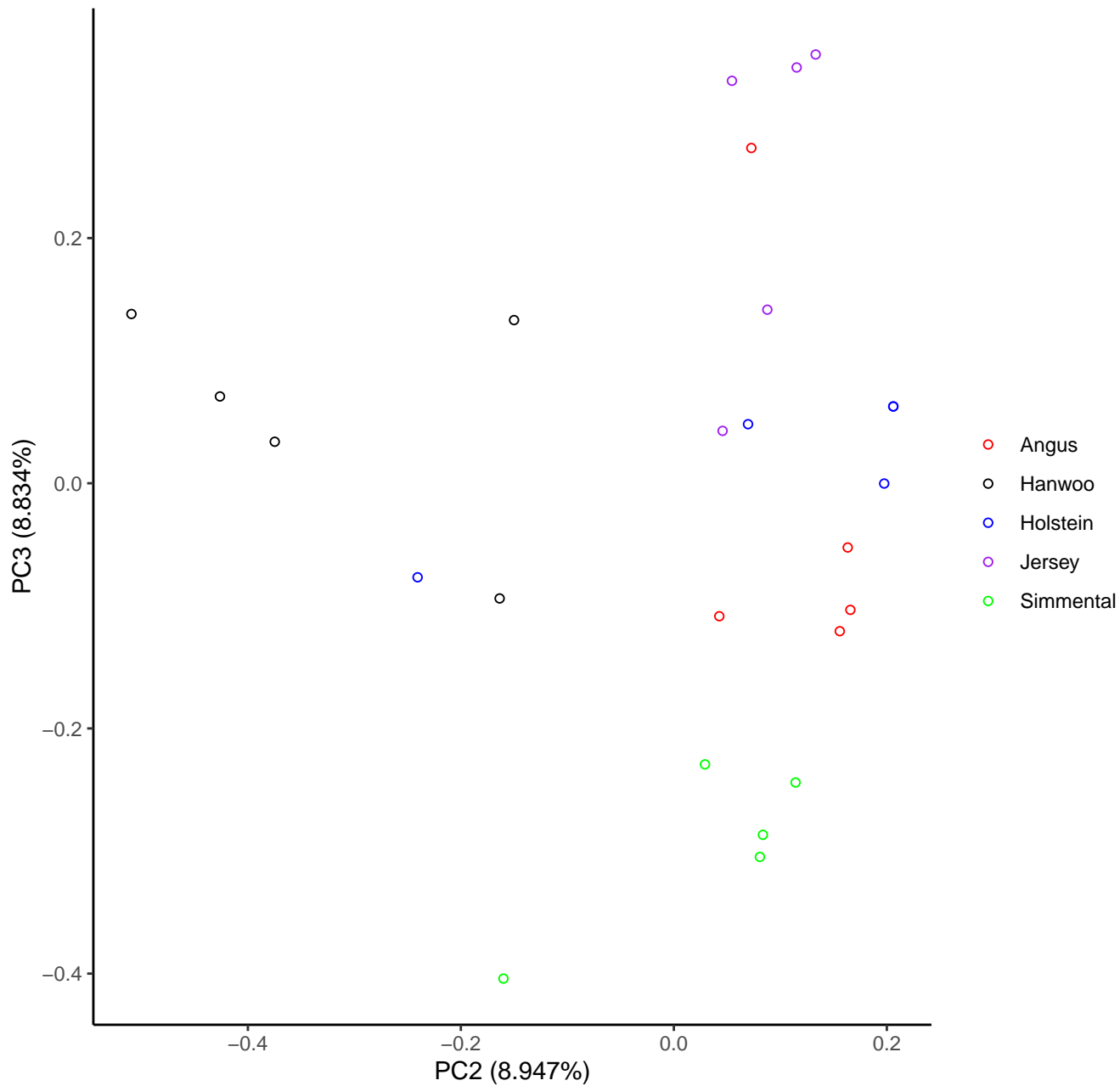
PCA analysis : 2-3
