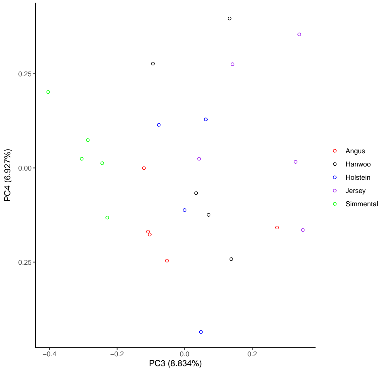
PCA analysis : 3–4
