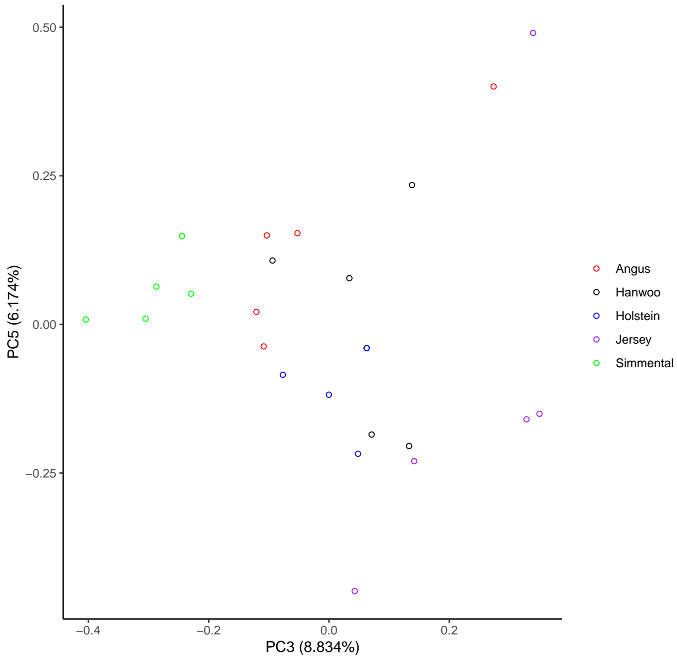
PCA analysis : 3–5
