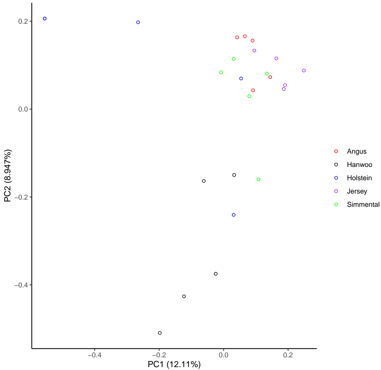
PCA analysis : 1-2
