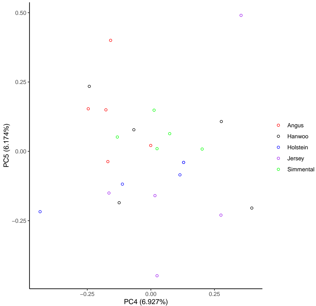
PCA analysis : 4-5
