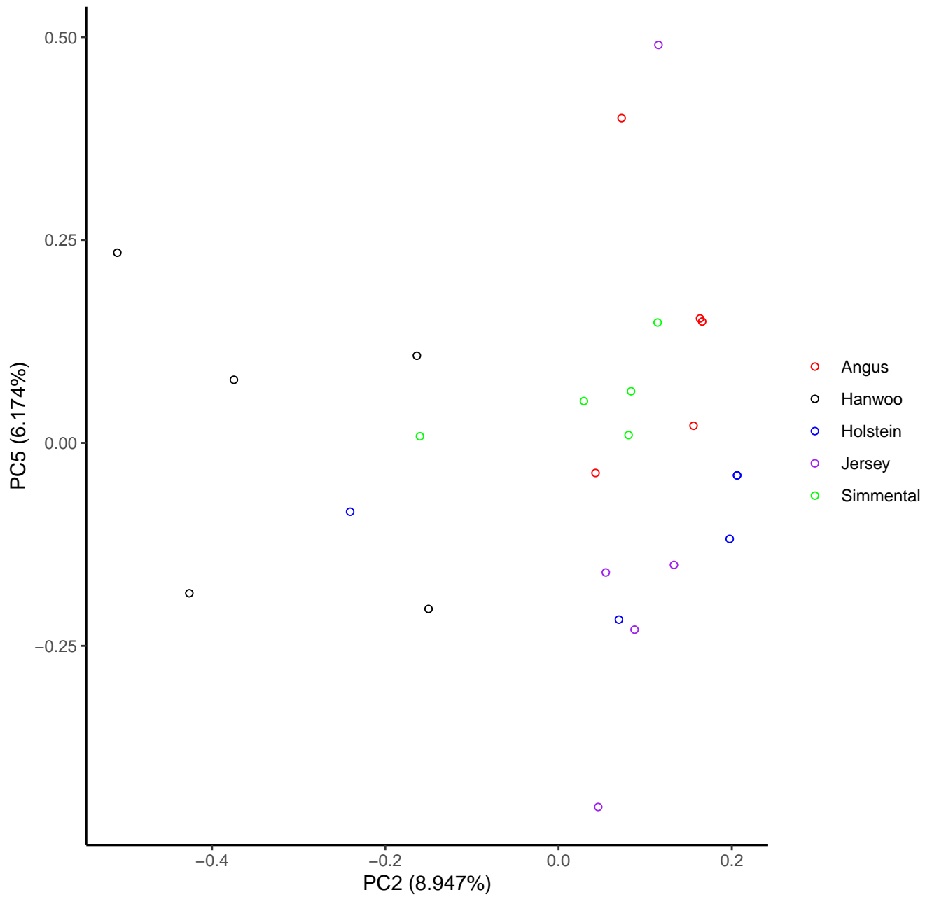
PCA analysis : 2-5
