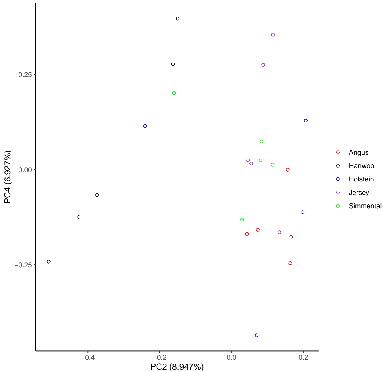
PCA analysis : 2-4
